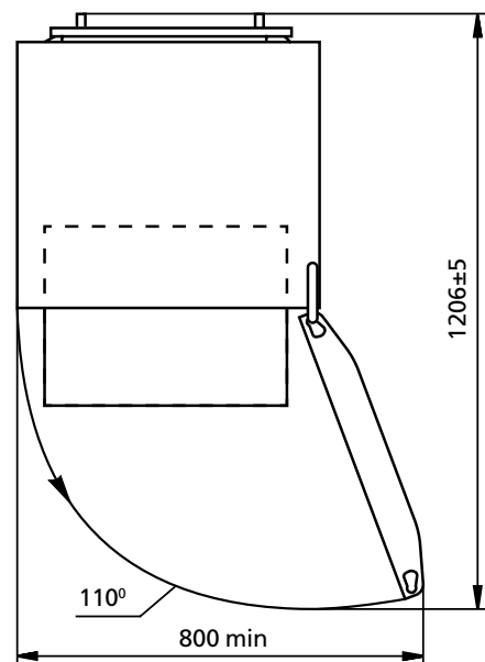
Рисунок 2 – Холодильник (вигляд зверху)
