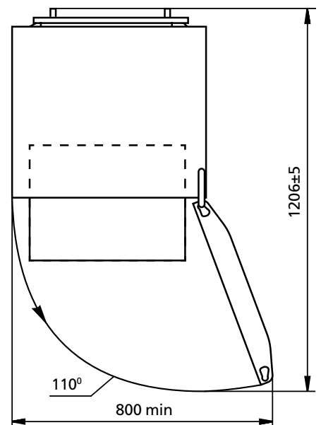
Тасвири 2 — Яхдон (намо аз боло)
