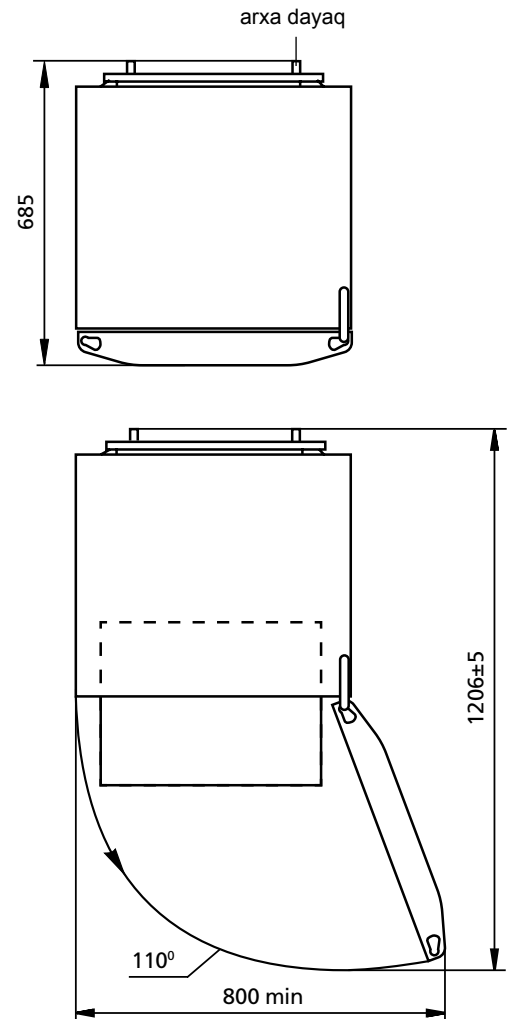
Şəkil 2 — Soyuducu (üstdən görünüşü)
